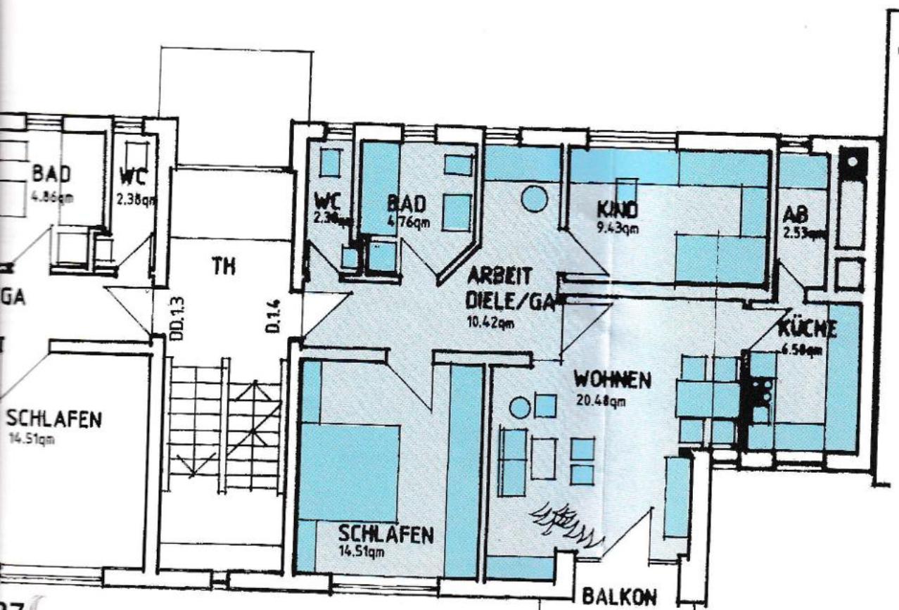
WOHNUNG 36 DIN 71.84 qm
