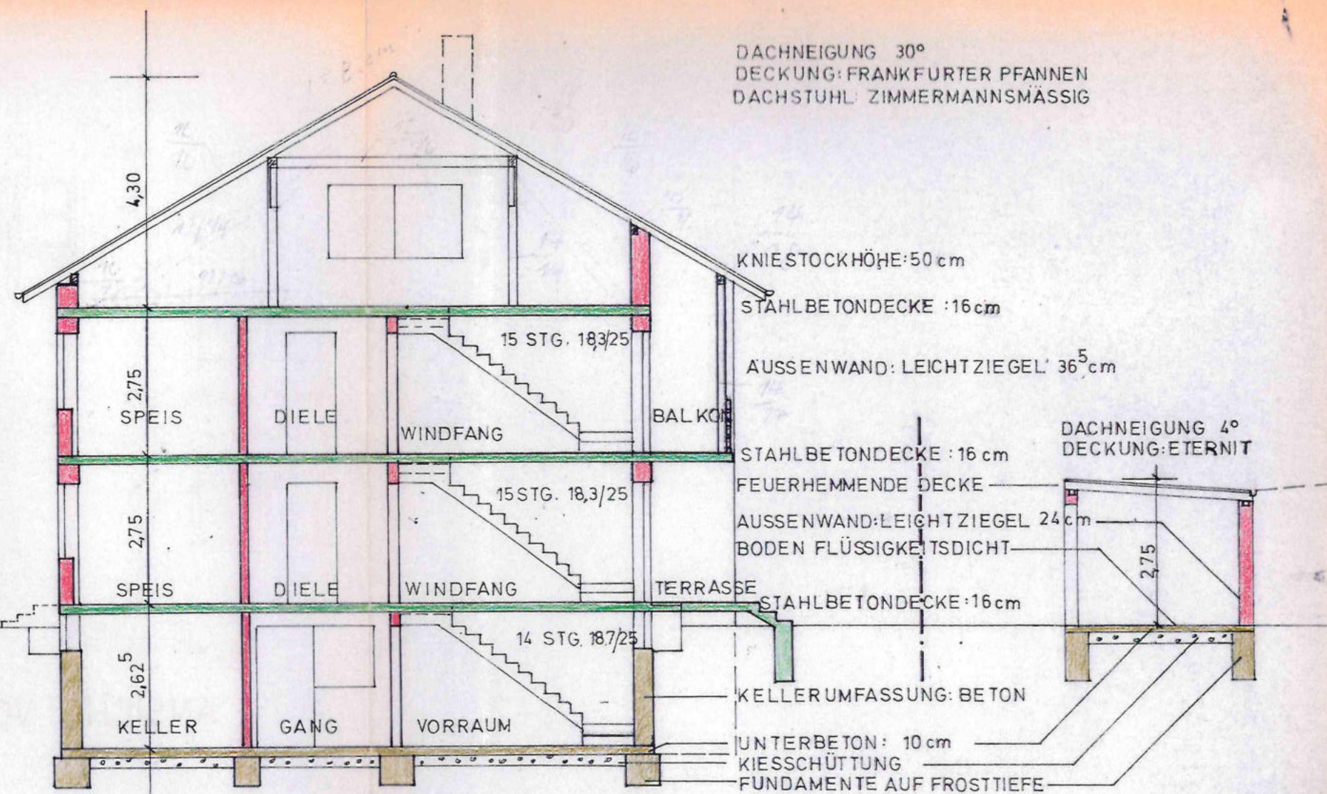
SCHNITT B-B'
