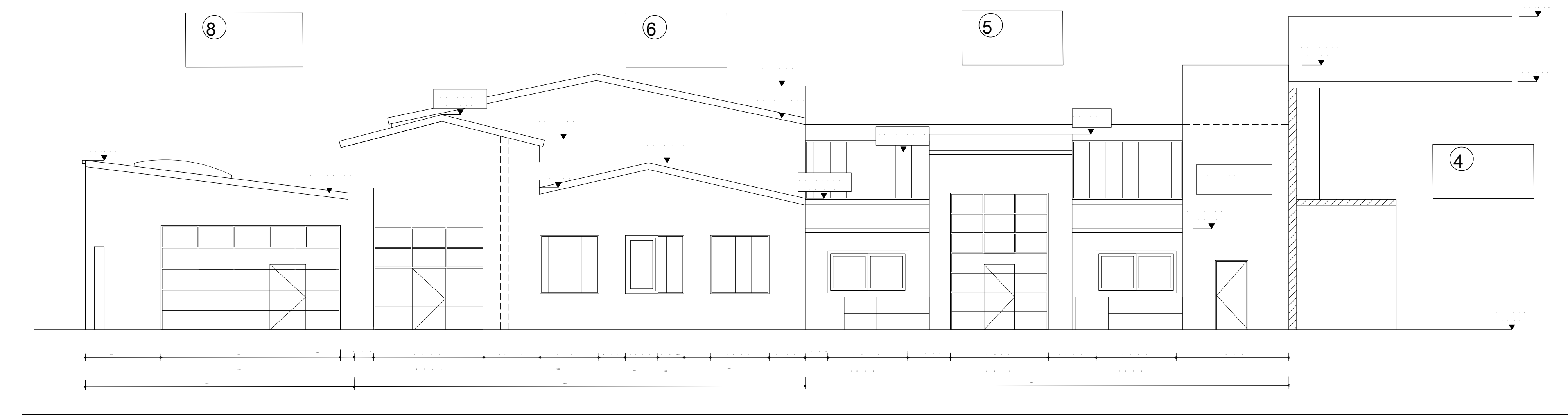
SCHNITT C-C M 1:100
