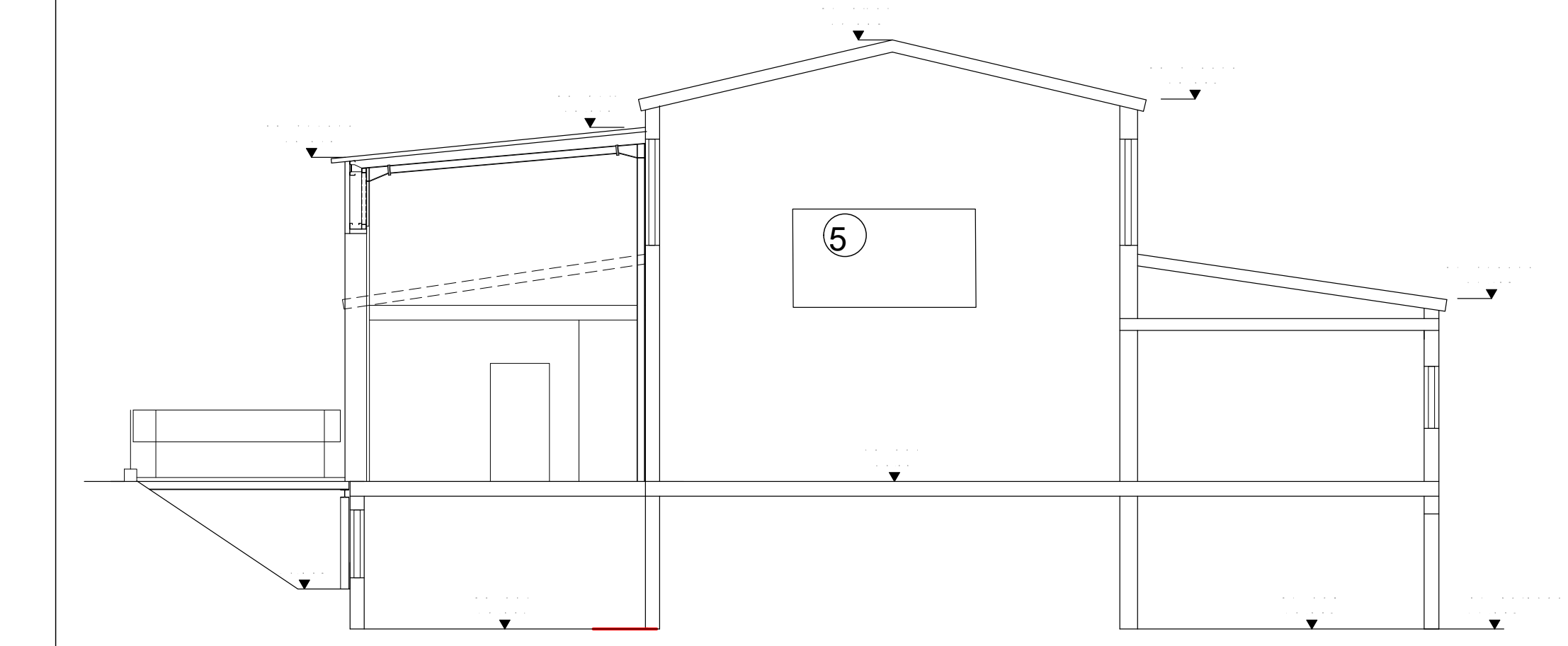
SCHNITT D-D M 1:100
