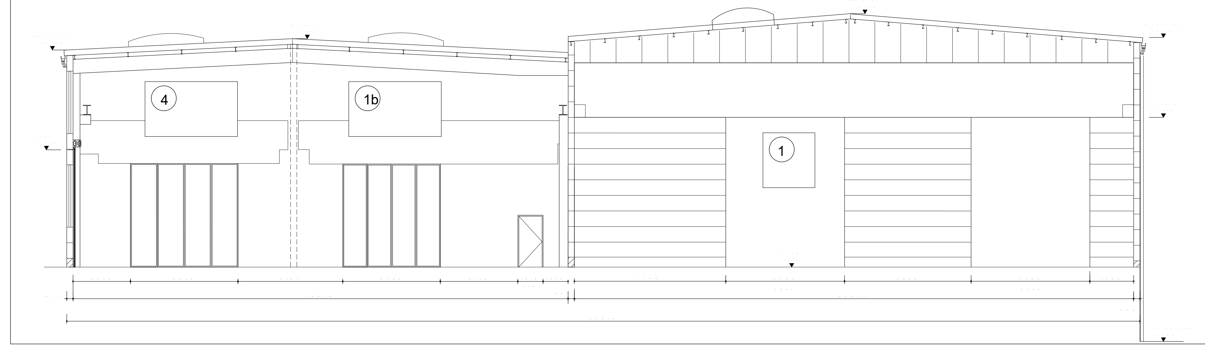
SCHNITT A-A M 1:100
